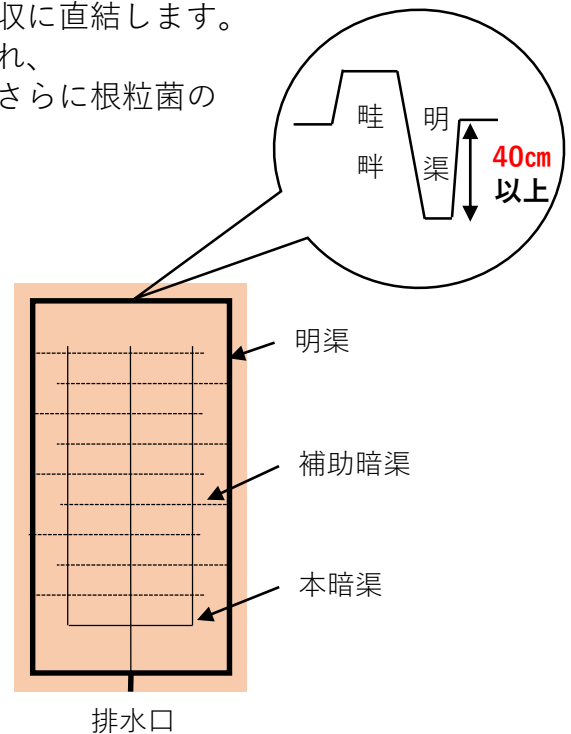
図1 明渠と補助暗渠の施工例
